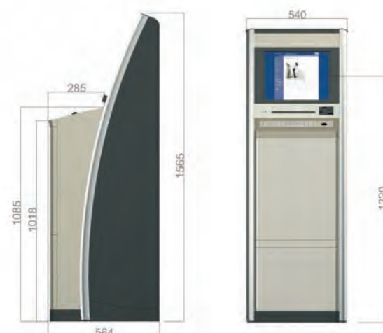
Smart Kiosk F103
